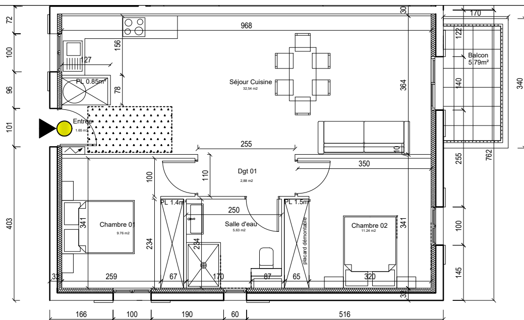
BATIMENT N°04 APPART N°411 PLAN REZ DE CHAUSSEE Echelle: 1/100 ème
