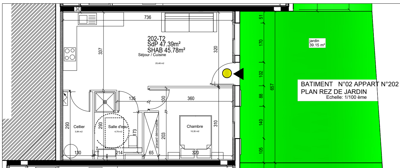
BATIMENT N°02 APPART PLAN REZ DE JARDIN Echelle: 1/100 ème
